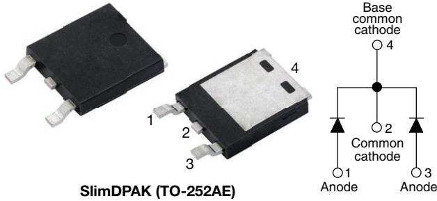
SlimDPAK (TO-252AE)
