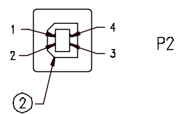
USB B Receptacle
