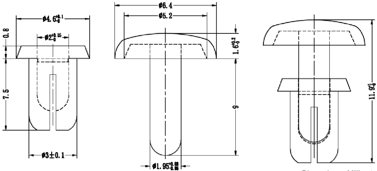
Dimensions : Millimetres
