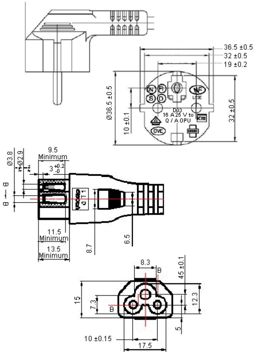
Dimensions : Millimetres
