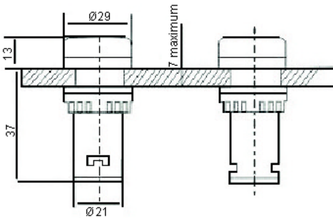
Dimensions : Millimetres
