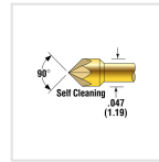
POGO-1Z1-S
