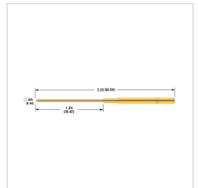
LTR-1W-2LL
