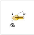
POGO-1T-S
