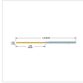
ELTR-1W-2LL
