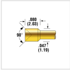
POGO-1L18
