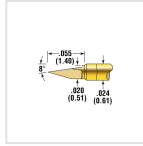
POGO-1B-S
