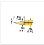
POGO-1Z-S
