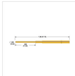
LTR-1W-2L
