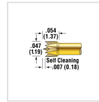
POGO-1V-S
