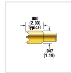
POGO-1L24-S
