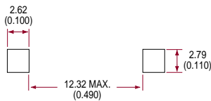
Mini-DYAD™ SMT
