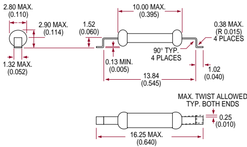
Mini-DYAD™ SMT
