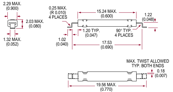
DYAD® SMT
