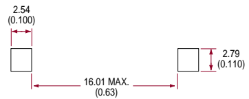
DYAD® SMT
