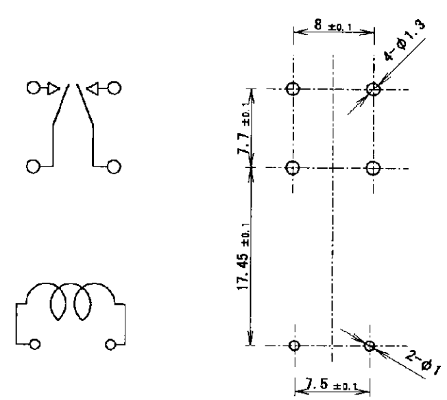
接続図 (2:1) フリット基板加工図 (2:1)
