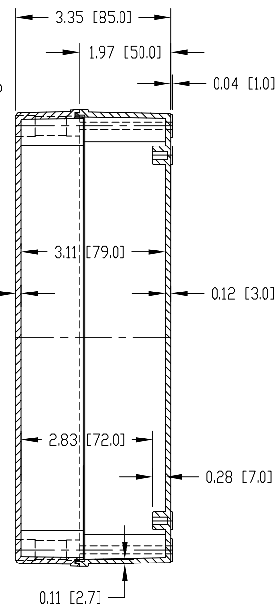
SECTION A-A
