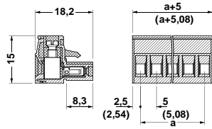
MSTB 2,5 HC/...-ST(-5,08)
