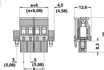
MVSTBW 2,5 HC/...-STF(-5,08)
