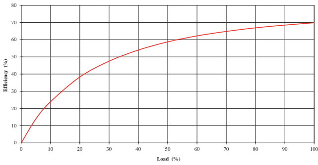
MGJ2D052005MPC
