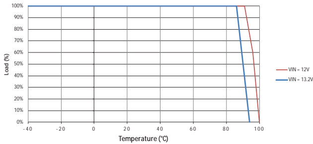
MGJ2D121509MPC
