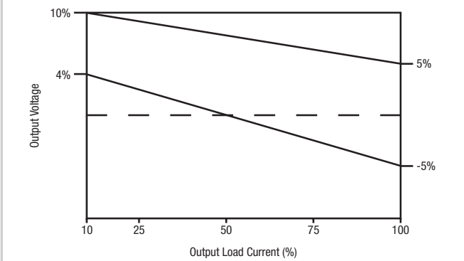
MGJ2D121509MPC
