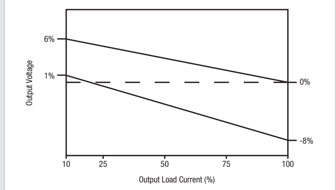
MGJ2D122005MPC
