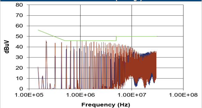
MGJ2D122005MPC (Average)
