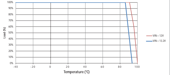
MGJ2D121505MPC
