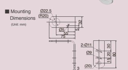
'L' Bracket Model: SZL-001
