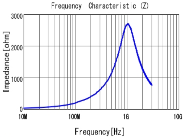
■ LQW18CAR33J00 |Z|
