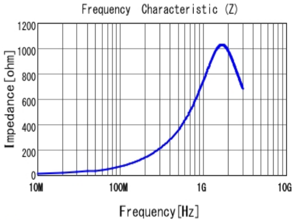
■ LQW18CAR12J00 |Z|
