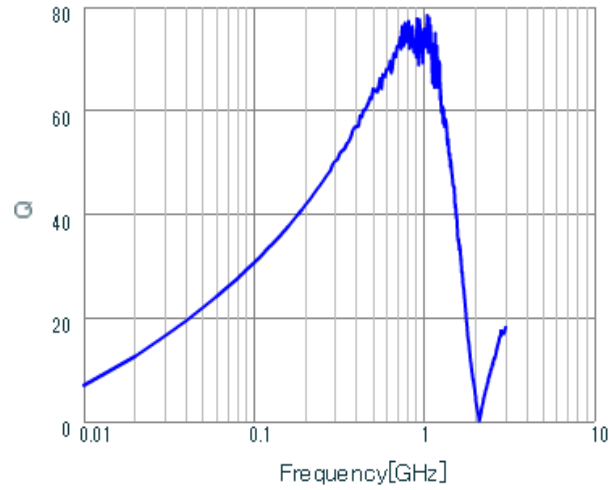
LQW18ANR12G00 Q.
