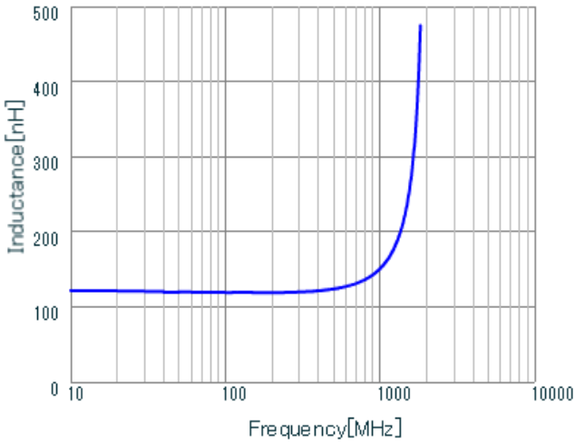
LQW18ANR12G00 L.
