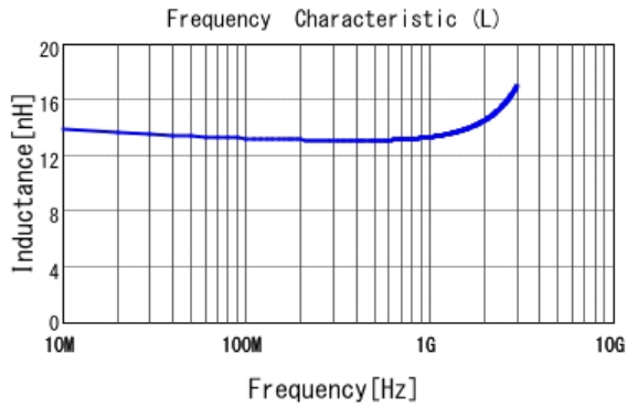
■ LQW18AN13NJ00 L
