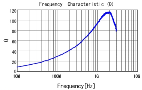
■ LQW18AN13NJ00 Q
