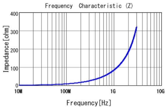
■ LQW18AN13NJ00 |Z|
