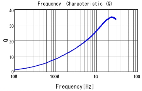
■ LQP03TN6N2H02 Q
