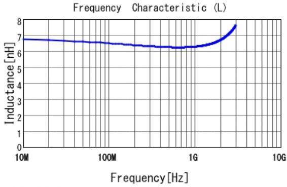
■ LQP03TN6N2H02 L
