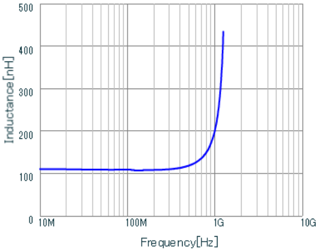
LQP03HQR11J02 L.
