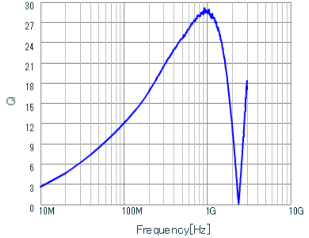
LQP03HQ39NH02 Q.
