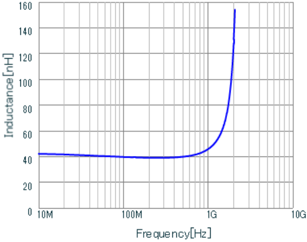
LQP03HQ39NH02 L.
