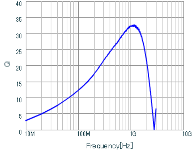
LQP03HQ30NH02 Q.
