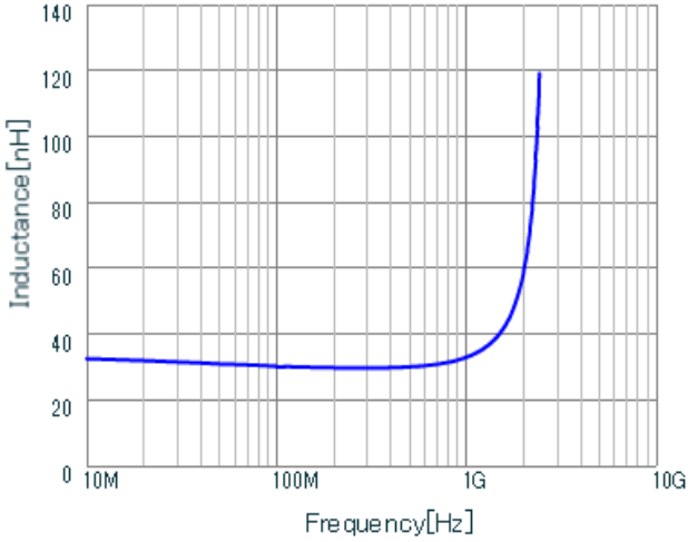
LQP03HQ30NH02 L.
