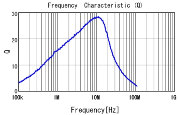
■ LQM2MPNR47NG0 Q
