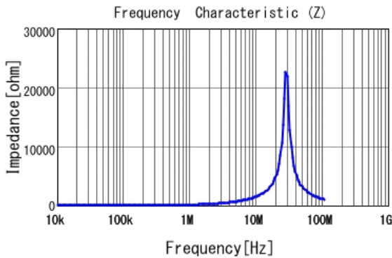
■ LQH2HPZ220MJR |Z|
