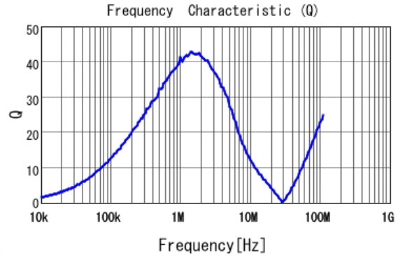
■ LQH2HPZ220MJR Q
