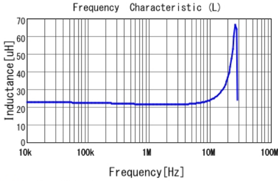
■ LQH2HPZ220MJR L
