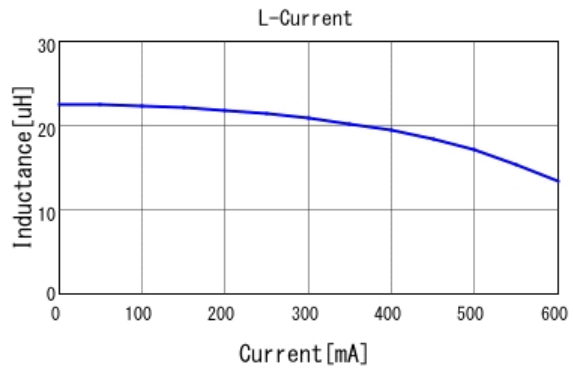
■ LQH2HPZ220MJR L-Current 20degC
