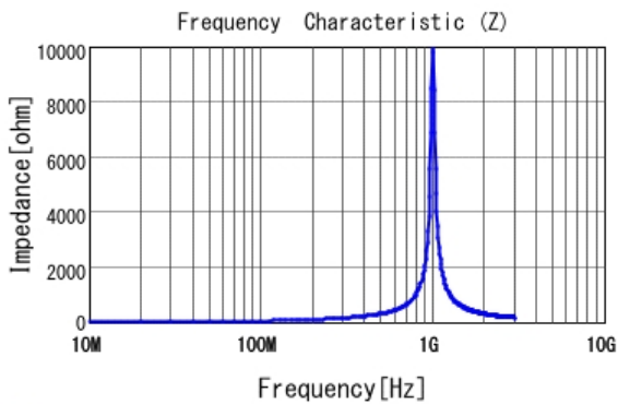
■ LQG15HS82NJ02 |Z|
