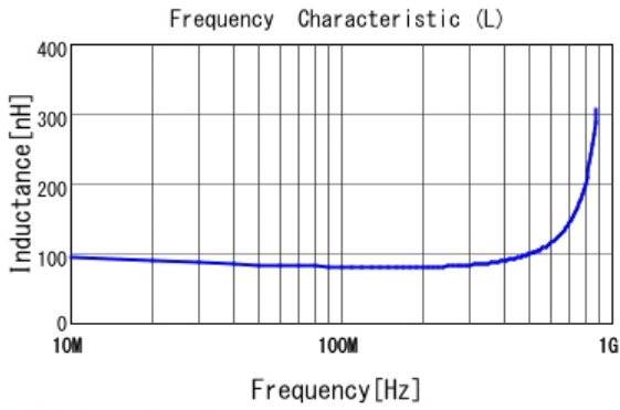
■ LQG15HS82NJ02 L
