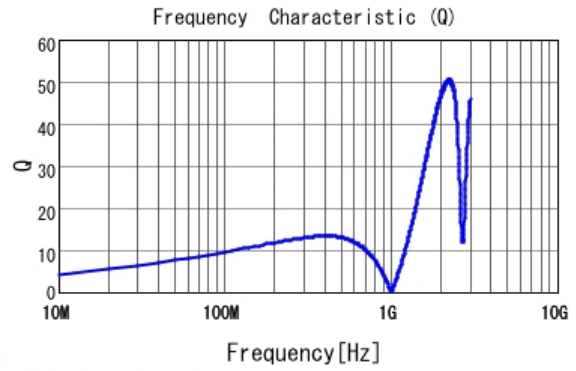
■ LQG15HS82NJ02 Q
