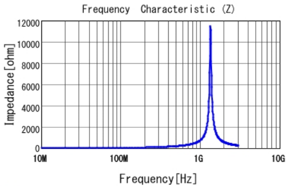
■ LQG15HS56NJ02 |Z|
