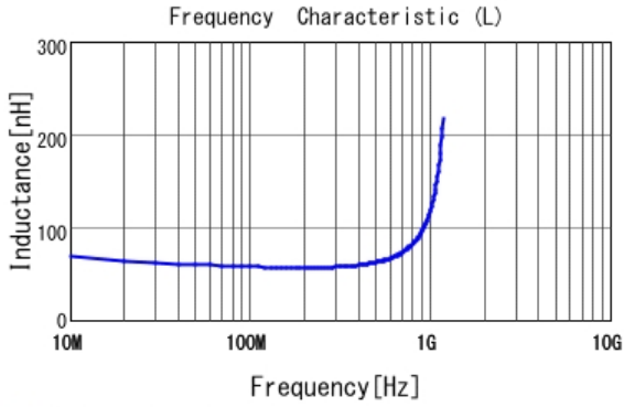
■ LQG15HS56NJ02 L
