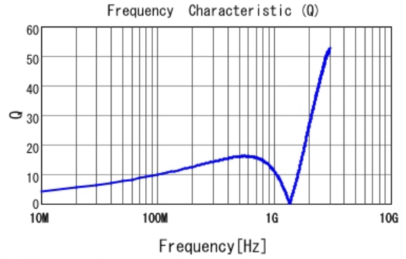
■ LQG15HS56NJ02 Q
