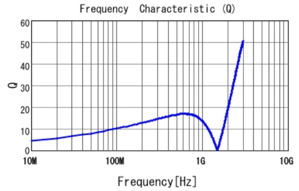
■ LQG15HS47NH02 Q
