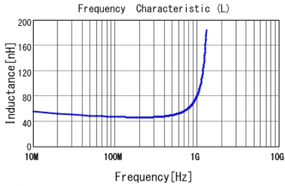
■ LQG15HS47NH02 L
