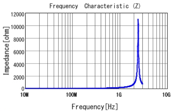
■ LQG15HS22NH02 |Z|
