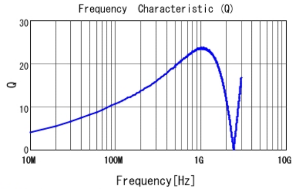
■ LQG15HS22NH02 Q
