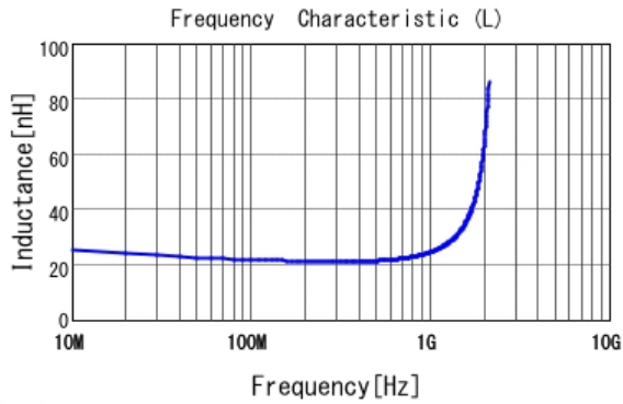
■ LQG15HS22NH02 L
