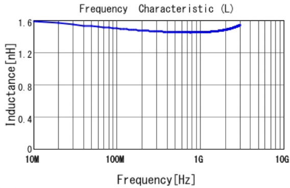
■ LQG15HN1N5C02 L
