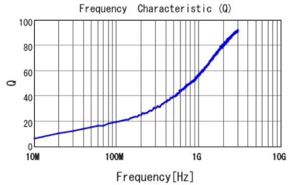
■ LQG15HN1N5C02 Q
