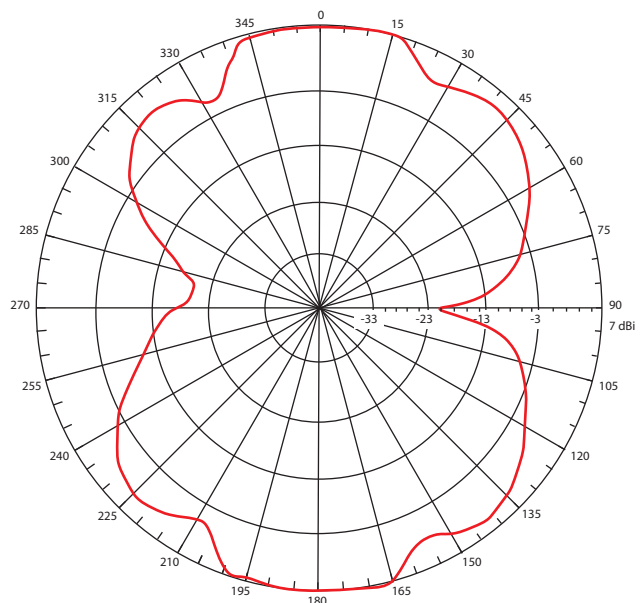
E-PLANE
