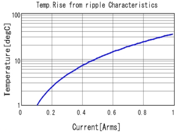
■ GRT033R60J104KE01 Temp. rise 800kHz
