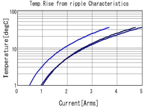
GRM31CR71E106KA12 Temp. rise ■ 80kHz ■ 400kHz ■ 800kHz
