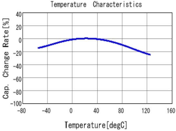
■ GRM188D71A106MA73 C-Temp. capchange, DCO. 0V, ACO. 2V rm
