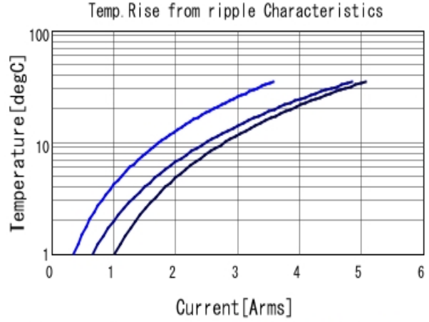
GRM188D71A106MA73 Temp. rise ■ 80kHz ■ 400kHz ■ 800kHz
