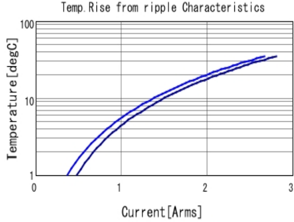
GRM033R60J225ME47 Temp. rise ■ 500kHz ■ 1MHz
