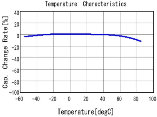
■ GRM033R60J225ME47 C-Temp. capchange, DCO. 0V, ACO. 2V rm
