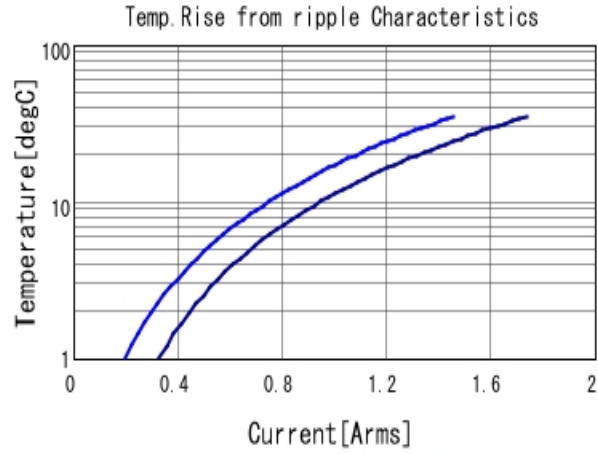
GRM033C80J224KE90 Temp. rise ■ 600kHz ■ 1MHz
