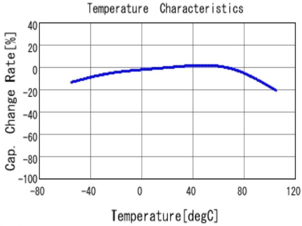
■ GRM033C80J224KE90 C-Temp. capchange, DCO. 0V, ACO. 1V rm
