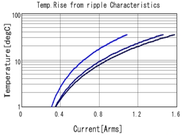
GCJ188R71C104KA01 Temp. rise ■ 400kHz ■ 800kHz ■ 1MHz
