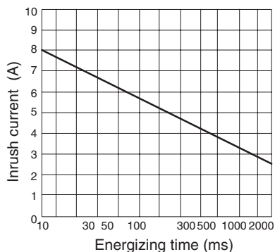
G3R-ODX025N
