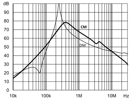
FN 3287-160-40-C33-R65
