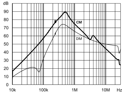
FN 3287-80-34-C33-R65
