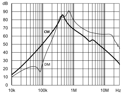
FN 3287-125-35-C33-R65
