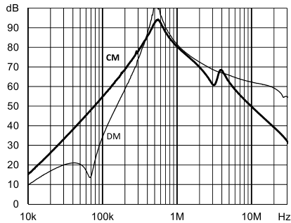
FN 3287-63-53-C33-R65
