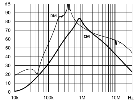
FN 3288-100-35-C21-R65
