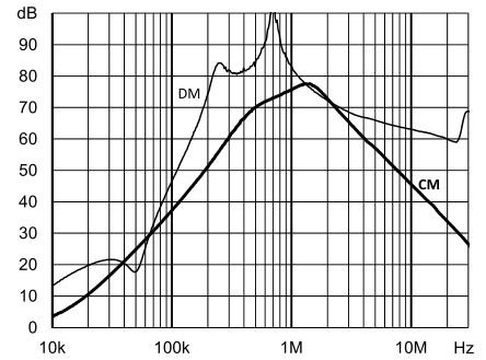
FN 3288-50-53-C21-R65
