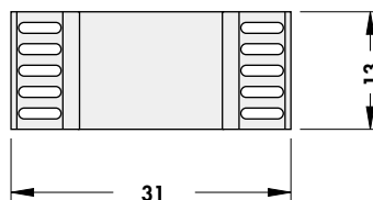
Gewicht/weight/poids: 3,6 g
