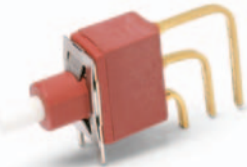
E112SD1AV2BE SPDT
