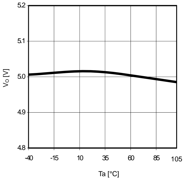
Figure 21. Ta-V O (I O =0mA)
