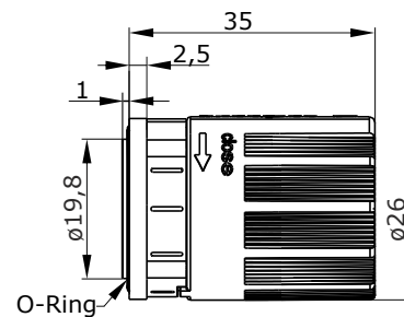
Hauptabmessungen Durchführung
