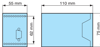
Modem
