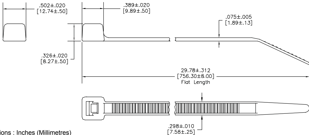
Dimensions : Inches (Millimetres)
