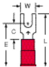
MV18-6FB/S Stud Size: 6 Wire Range: 22-18
