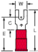
MV18-4FB/S Stud Size: 4 Wire Range: 22-18
