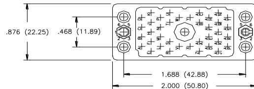
56 PIN RECEPTACLE
