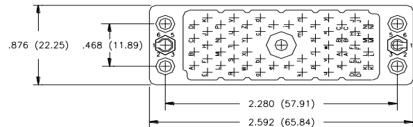
90 PIN RECEPTACLE
