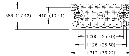
20 PIN RECEPTACLE
