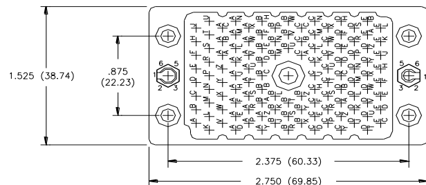
120 PIN RECEPTACLE
