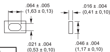
SOLDER LUG TERMINAL DETAIL 22.5°
