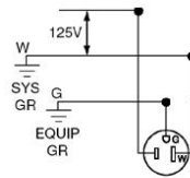
5-15R
