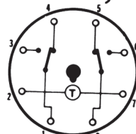
TERMINAL WIRING
