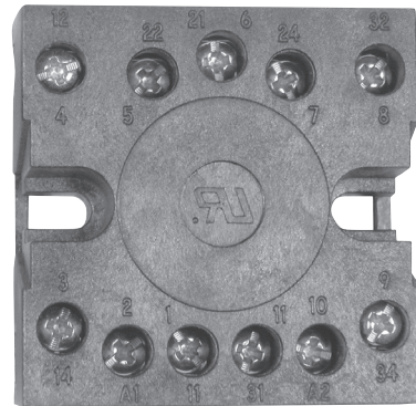
600-3-0012 Panel Mount, 11 Pin 47mm (W) x 47mm (T) x 20mm (D)
