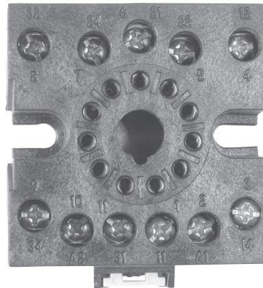
600-3-0014 DIN Rail or Base Mount, 11 Pin 47mm (W) x 47mm (T) x 20mm (D)
