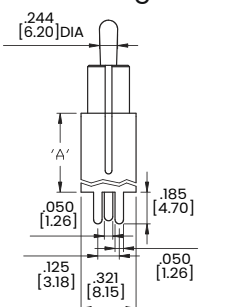
VS2-VS3 Single Pole
